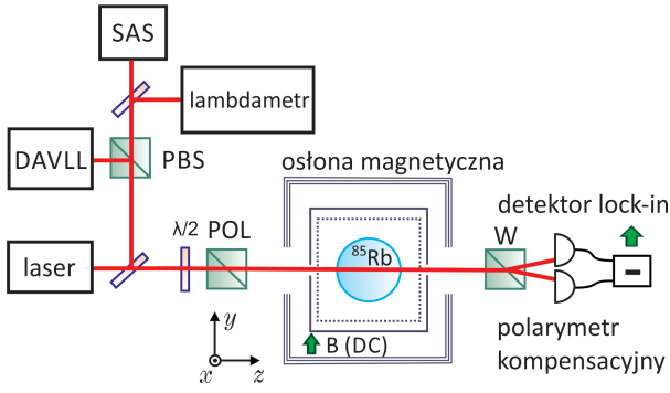
Rysunek 1: Schemat układu doświadczenia. Poszczególne skróty oznaczają: DAVL – stabilizator długości fali światła laserowego, SAS – nasyceniowa spektroskopia absorpcyjna, PBS – polaryzacyjna kostka światłodzielająca, W – pryzmat Wollastona, \lambda/2 – płytka półfalowa używana razem z polaryzatorem Glana-Thompsona (POL) do regulacji natężenia światła. Sygnały informujące o skręceniu polaryzacji są rejestrowane za pomocą komputera (nie zamieszczony na schemacie).
